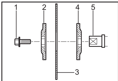
► 1. Tornillo hexagonal 2. Brida exterior 3. Disco de sierra 4. Brida interior 5. Eje
