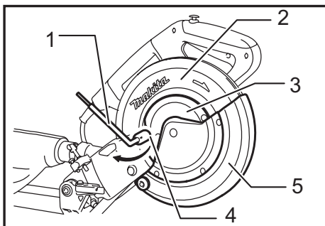
► 1. Llave de cubo 2. Caja del disco 3. Cubierta central 4. Tornillo hexagonal 5. Protector de disco
