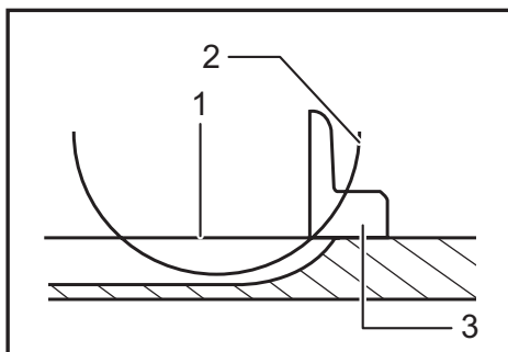
► 1. Parte superior de la base giratoria 2. Perifería del disco 3. Guía lateral
