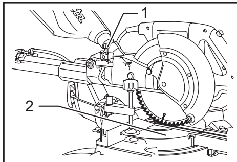
► 1. Perno de ajuste 2. Base giratoria
