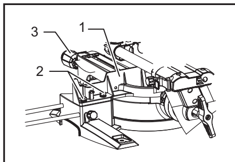
► 1. Guide fence 2. Hex bolts 3. Grip
