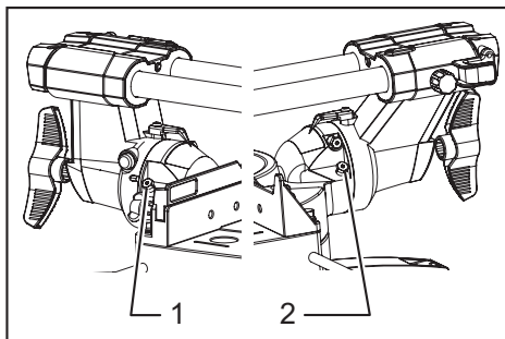
► 1. Boulon de réglage d'angle de biseau 5° droit 2. Boulon de réglage de l'angle de coupe en biseau 45° de gauche
