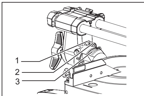
► 1. Tornillo 2. Apuntador o puntero 3. Escala de bisel
