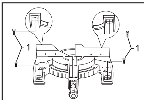
► 1. Pernos
