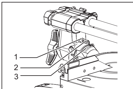
► 1. Vis 2. Index 3. Échelle de coupe en biseau
