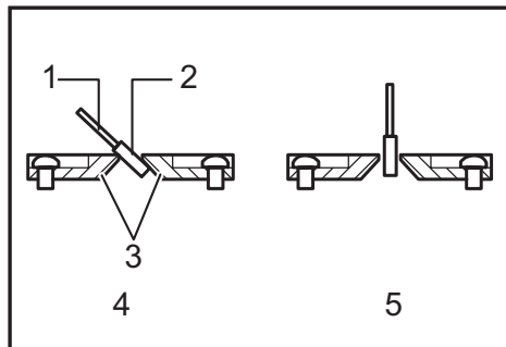
► 1. Lame 2. Dents de la lame 3. Plateau de découpe 4. Coupe en biseau sur la gauche 5. Coupe rectiligne
