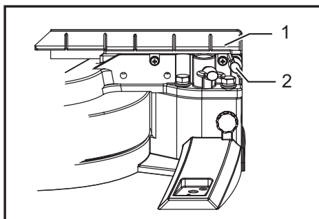
► 1. Guía de corte deslizable 2. Tornillo de fijación
