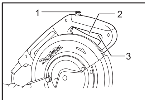
► 1. Botón lock-off (bloqueo desactivado) 2. Gatillo interruptor 3. Orificio para candado
