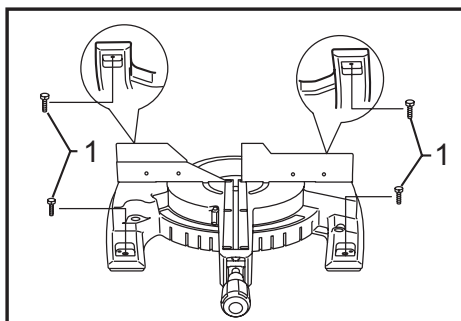
► 1. Bolts
