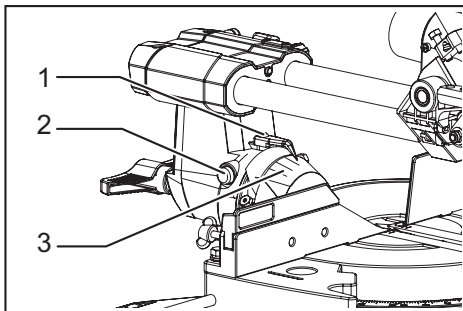
► 1. Apuntador o puntero 2. Botón de liberación 3. Escala de bisel
